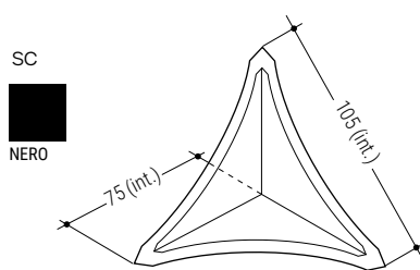
260 Salva angolo a tre vie con ammortizzatori d'urto 3-way corner protection Shock absorbers
