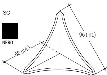
245 Salva angolo a tre vie 3-way corner protection
