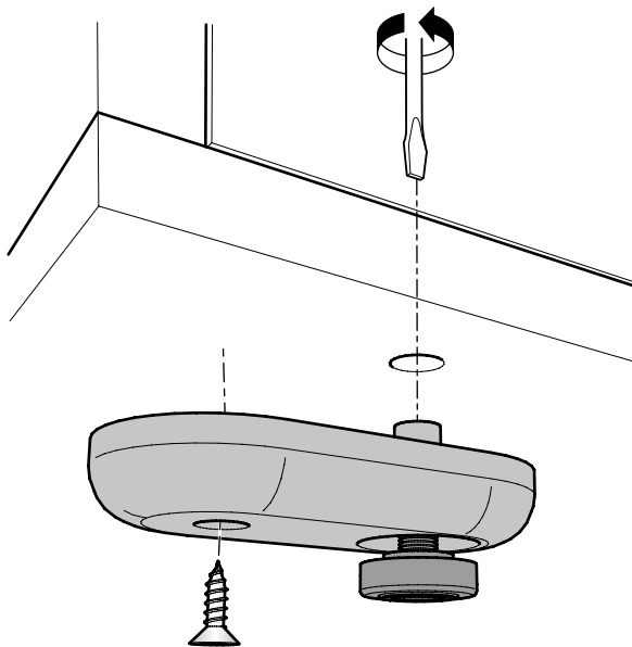
749 A Piedino regolabile h 27 mm Regolable bearing h 27 mm
