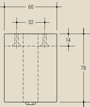
721R Regolabile / Adjustment 60x18 h 78 i. 32 flangia/flange 60x60 VE | VS | VG | MT | KU | SP
