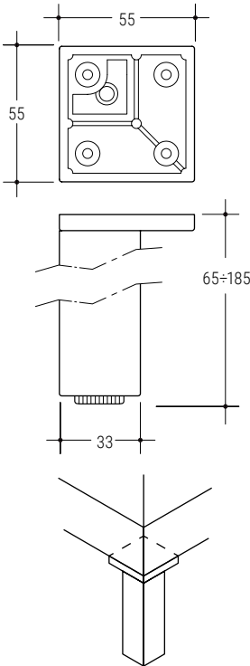
Piedino d'angolo Angle foot
