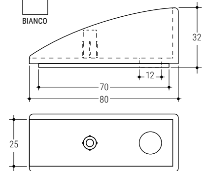
1777 B Tappo terminale gamba scrivania Desk leg end cap
