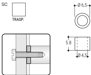
165 Rondella distanziatrice per vetri Spacer washer for glass 1000 Pz
