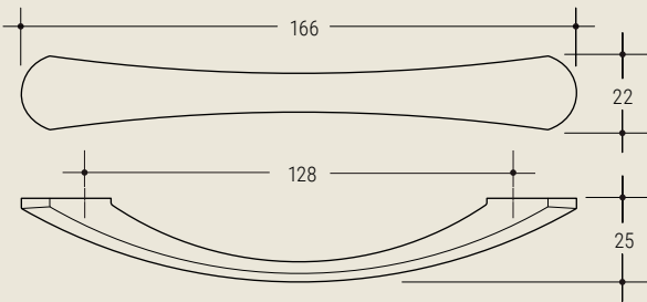
o91B 166x22 p 25 i 128 — VE | VS | VG | VA | VM | KU | SP
