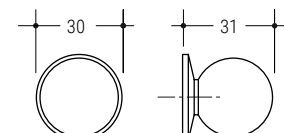
002 Ø 30 p 31 VE | VS | VG | VA | VM | VR | GA | KU | SP
