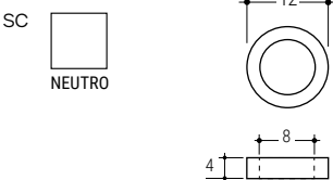
129 A Rondelle distanziatrici Washer-spacers 10000 Pz
