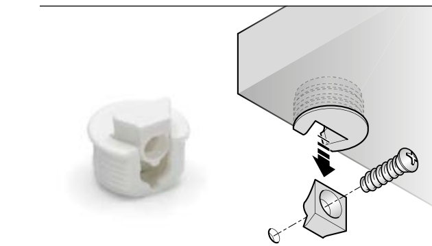
163 PL Reggipiano di unione per interparete Union-plan for interwall
