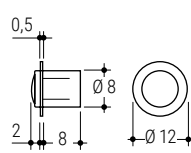
122 B Paracolpo ad incasso con battuta morbida Integrated bumper with soft edge 2500 Pz
