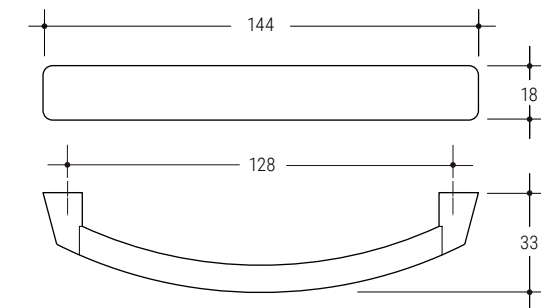
380 144x18 p 33 i 128 VE | VS | VG | VW | KU | SP VE | VS | VG | VM | SP
