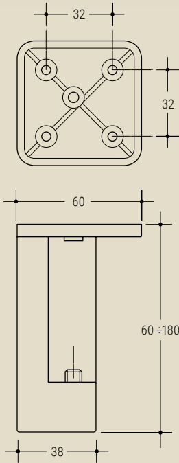
727R Regolabile / Adjustment 38x38 flangia/flange 60x60 h 60-180 VE | VS | VG | MT | SP
