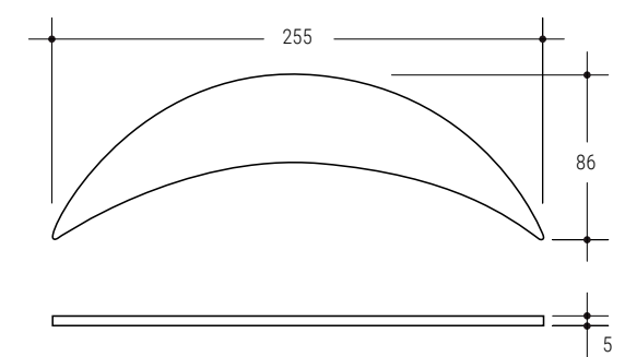
1669 Fissaggio con biadesivo Fixing with biadesive 255x86 VE | VS | VG | VR
