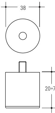
145AR Filetto 8MA anche sotto Screw 8MA in the bottom
