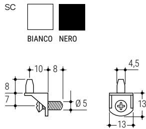
108 Reggipiano con vite ad espansione Bracket with expansion screw
