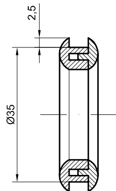
sez. A-A
