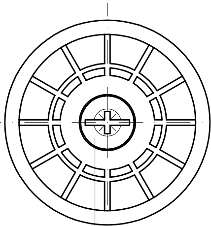
Vite TBL M8x35 Zn
