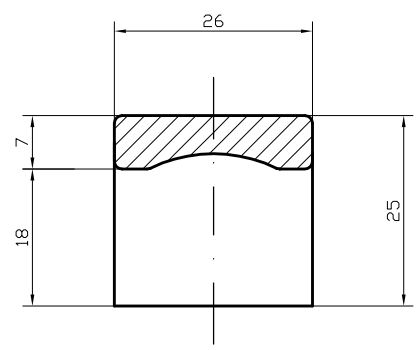
sez. A-A
